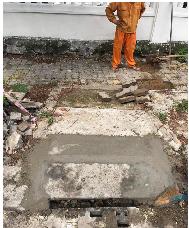
Hình ảnh sau xử lý tại các vị trí đan hư hỏng trên đường Dũng Sĩ Thanh Khê
